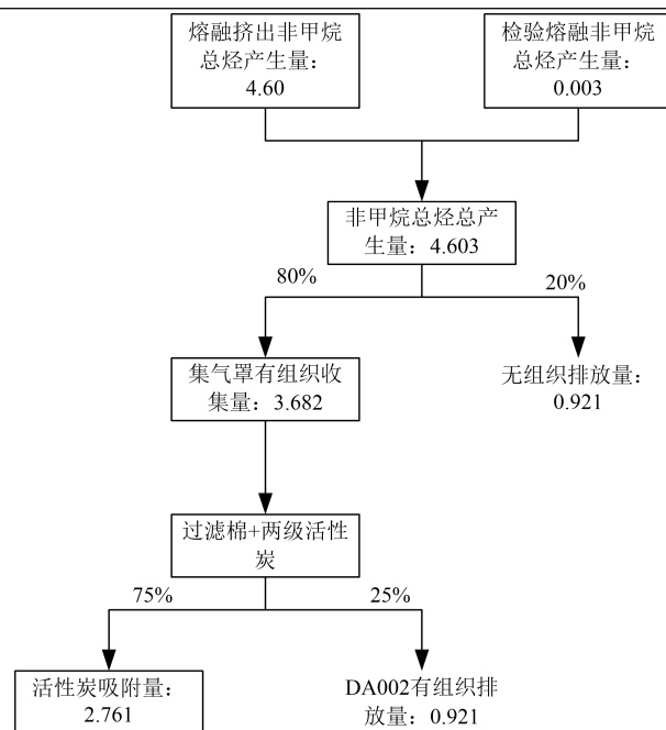
图 2.7-1 项目非甲烷总烃平衡图 单位: t/a
