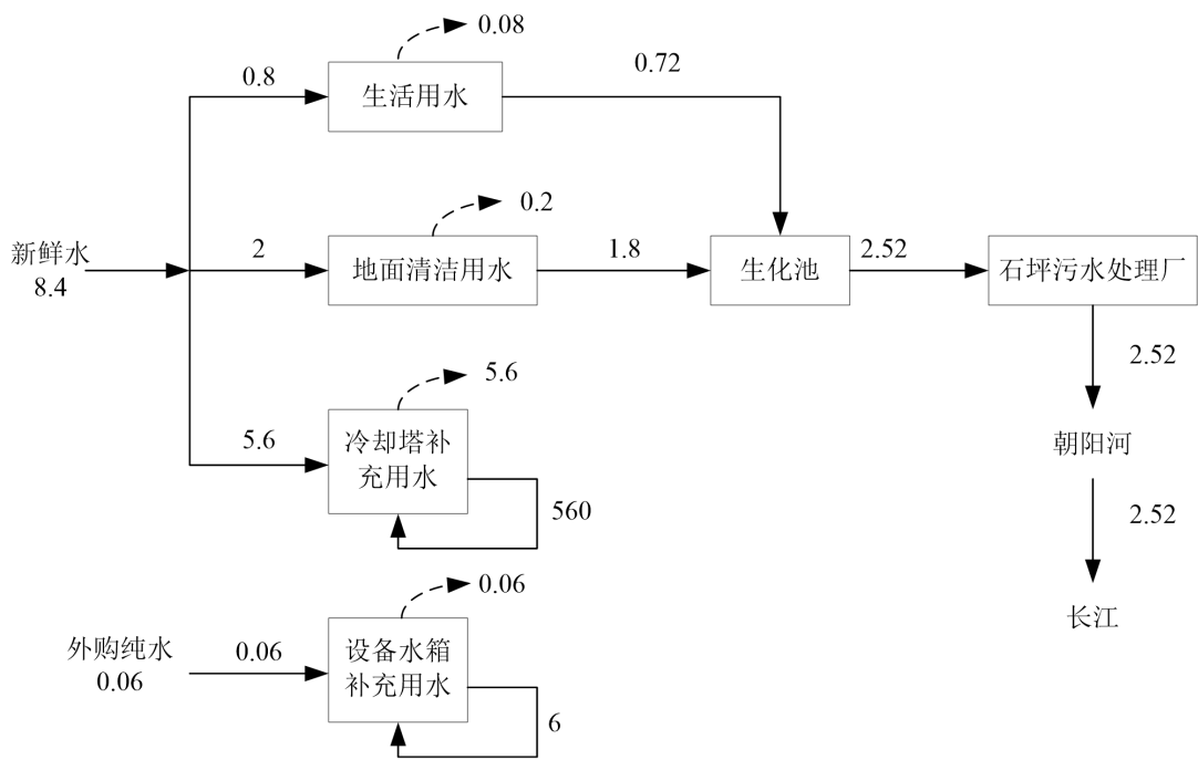
图 2.9-1 项目最大日排水水平衡图（单位：m 3 /d）
