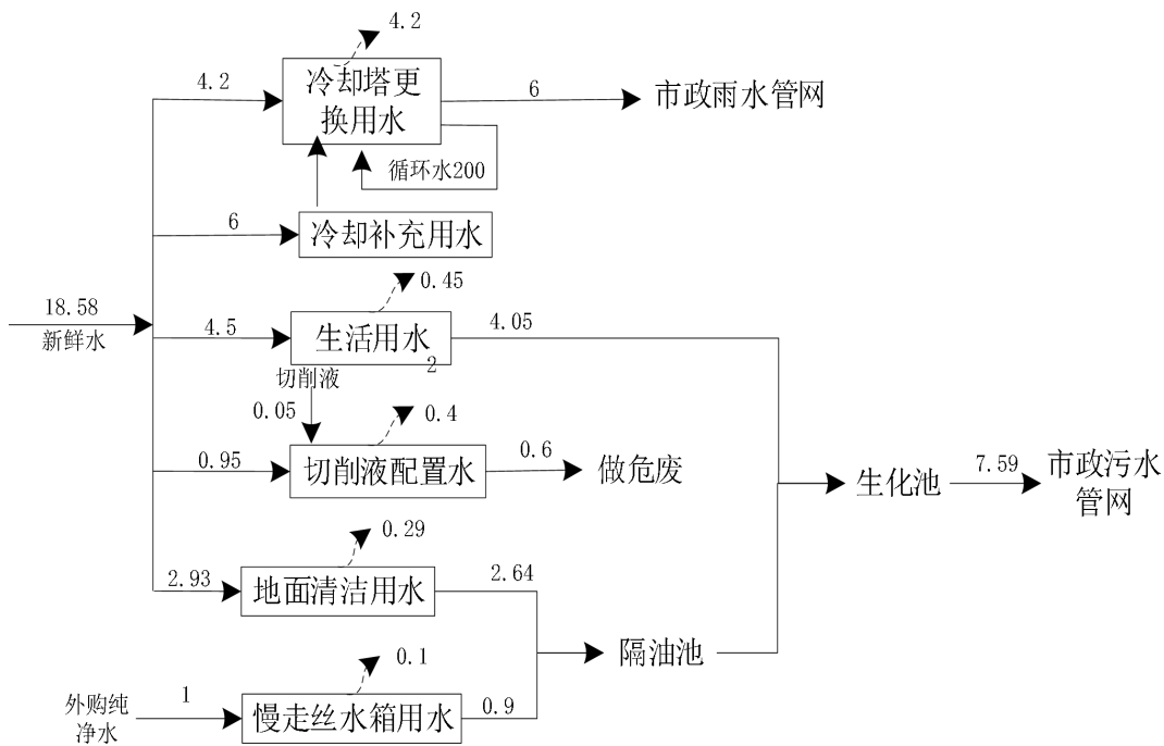
水平衡图：
