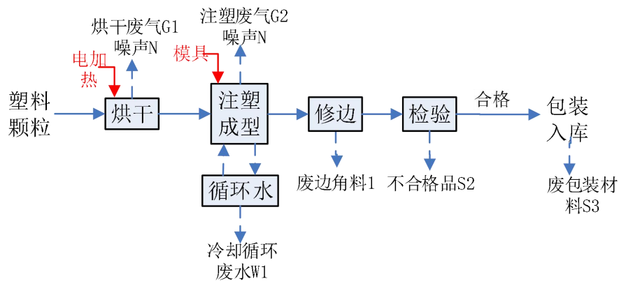
图 2-2 注塑件工艺流程图及主要产污环节
