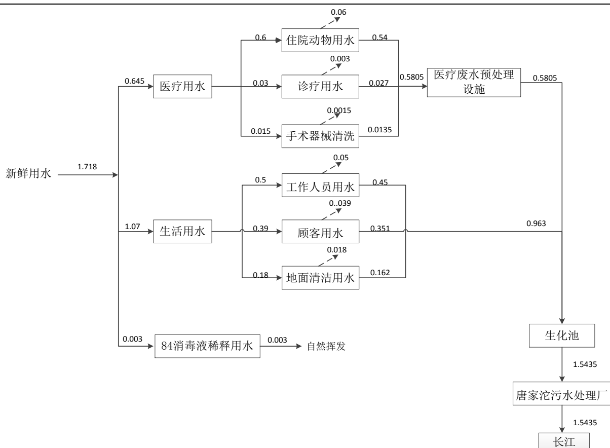
图 2-1 项目水平衡图 (单位: \text{m}^3/\text{d} )
