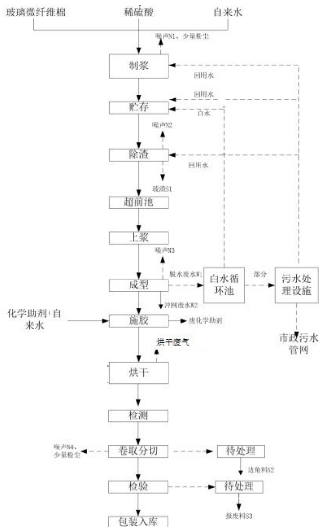
图 2.13-1 现有工程工艺流程及产污环节图
