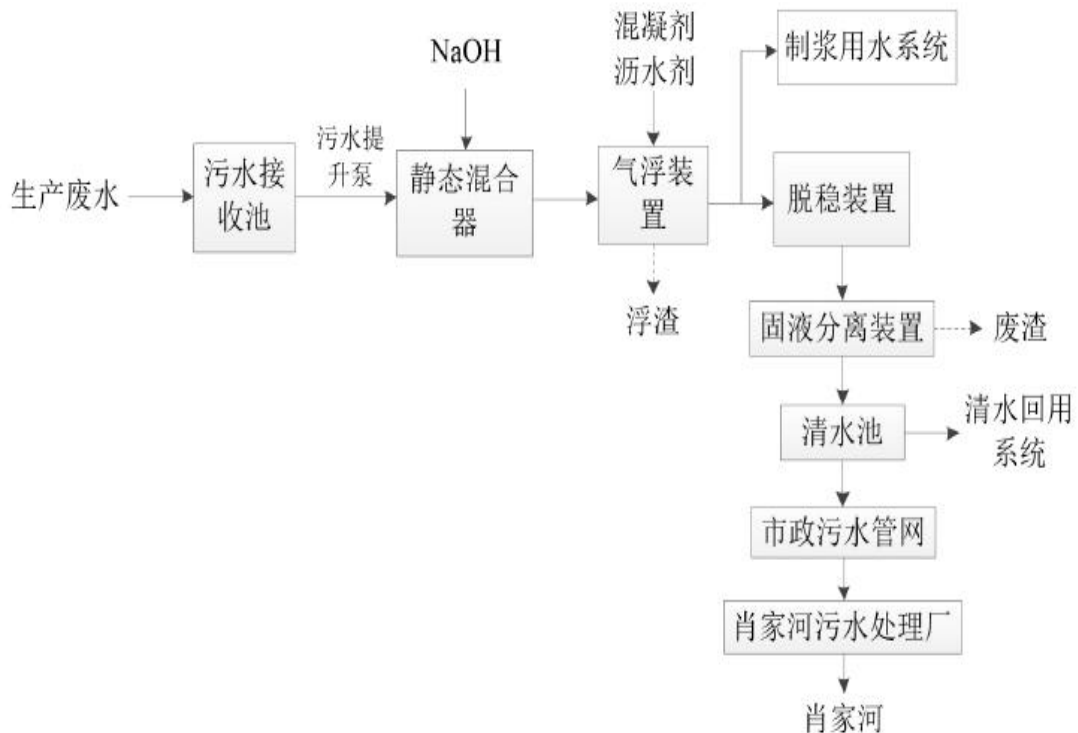
图 4.2-1 一体化污水处理设施工艺流程图
