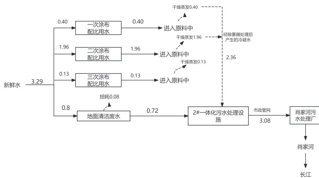
图 2.9-1 扩建项目水平衡图 (m³/d)
