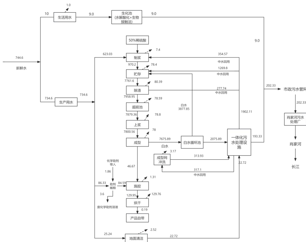
图 2.13-1 现有工程全厂水平衡图 (m 3 /d)
