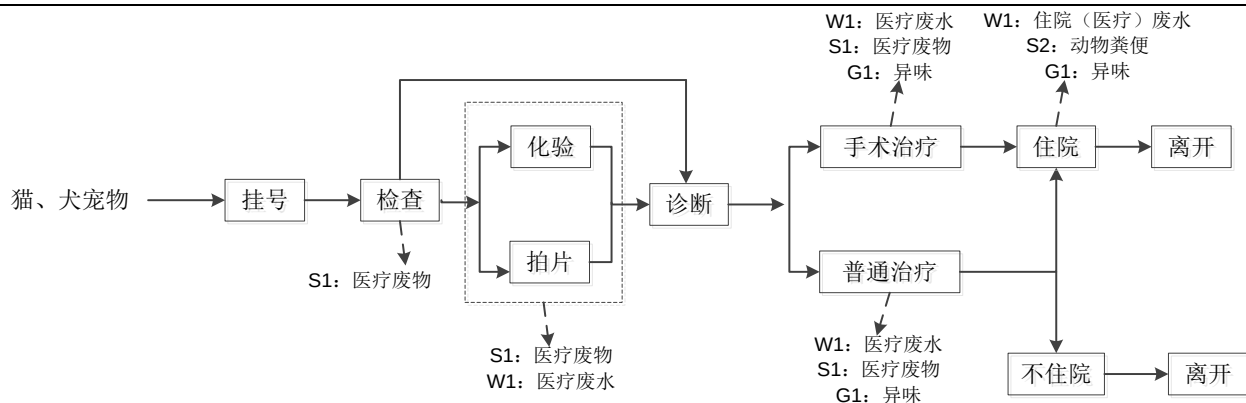
图 2-2 运营期宠物医院服务流程及产污环节图
