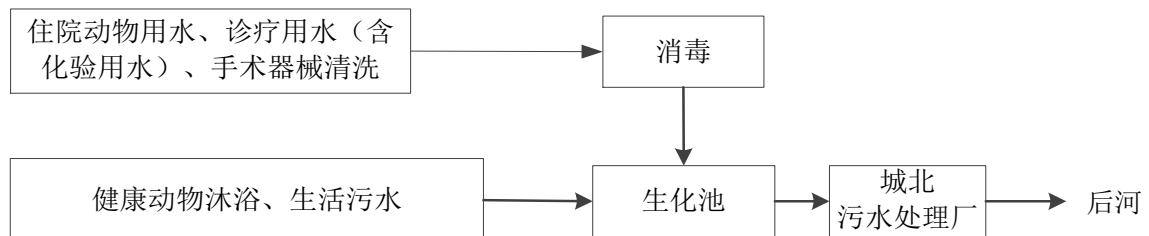
图 4-2 废水处理流程图
