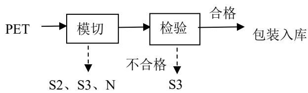
图2.3 铁电池隔板生产工艺流程及产排污示意图
