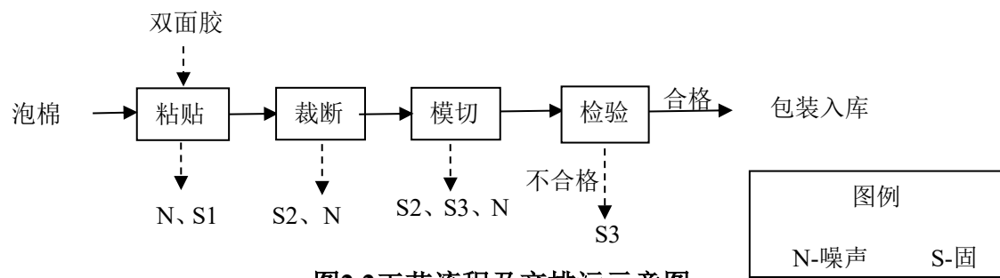
图2.2工艺流程及产排污示意图
