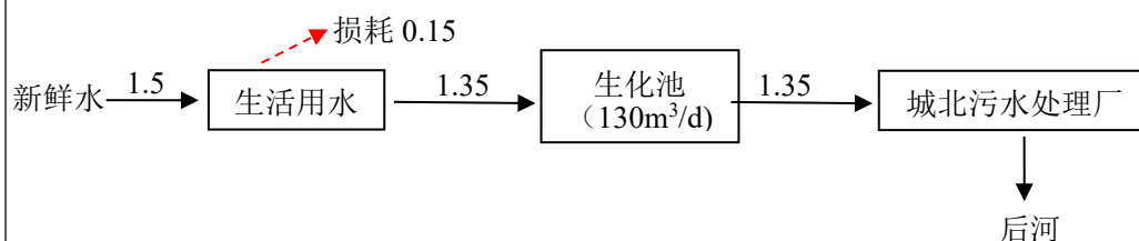
图 4.1 本项目水平衡图 单位：m³/d
